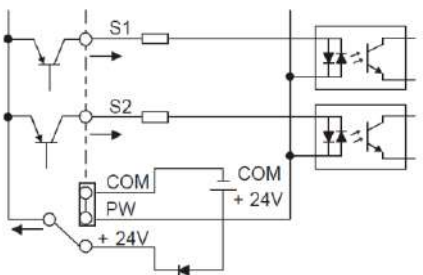
Внутреннее питание (PNP режим)
